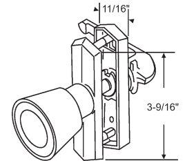
Tulip Knob Latch
