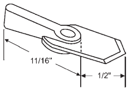
Part # Color 900-9823 Black 900-9823W White 900-9823N Natural
