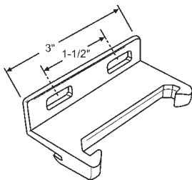
900-69 Die Cast Yale Ogron
