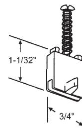
900-84 Bottom Guide Tucker
