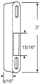
900-8856 Die Cast Keeper for 900-9169
