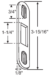
12-272 Flat. For 13-247 & 13-248 Patio Door Handles
