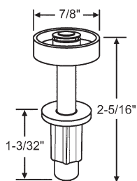
2-142 Guide Pin
