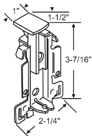
900-12459 Top Guide
