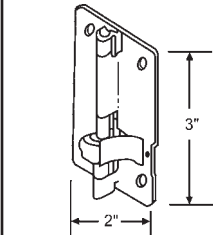
8-230 Door Hinge Paniflex
