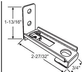
7-278 Pivot L-Bracket
