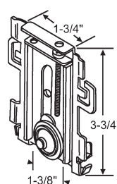
900-11827 Bottom Roller
