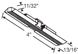
2-92 Pivot Guide Stanley
