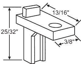
83-535 Pivot Bar
