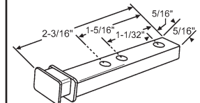
83-517 Pivot Bar
