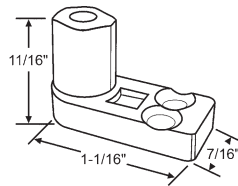
83-529 White
