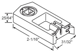
83-506
