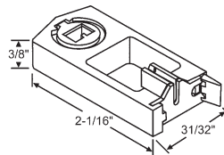
83-508
