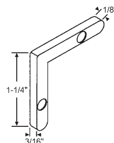
900-479 Die Cast
