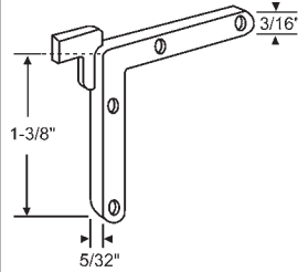
46-7 Die Cast
