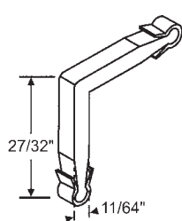
46-124 Die Cast
