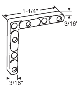
900-481 Die Cast
