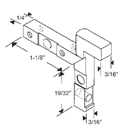
900-19068 Die Cast
