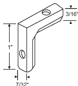
46-12 Die Cast
