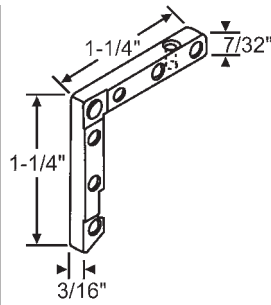
46-120 Die Cast
