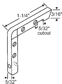
900-11892 Metal
