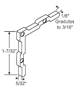
900-11008 Metal
