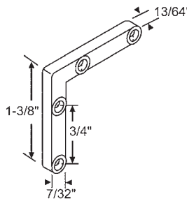
900-21287 Die Cast
