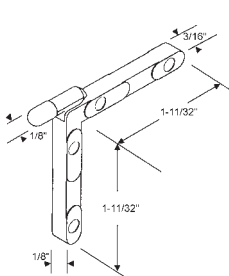
900-464 Die Cast
