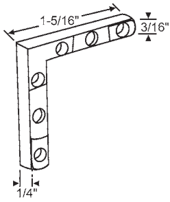
46-86 Die Cast
