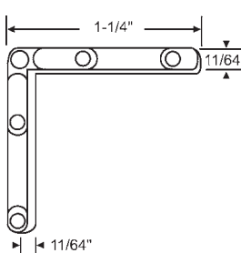
900-15214 Die Cast
